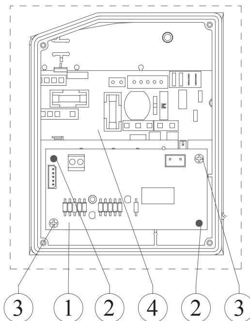
1. ábra: a relépanel telepítése
