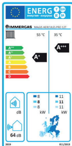
MAGIS HERCULES PRO 12T
