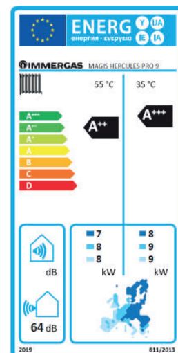
MAGIS HERCULES PRO 9
