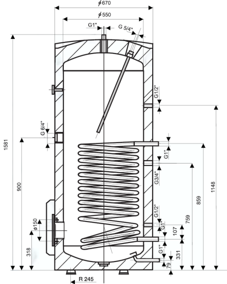
UBS 300 indirekt HMV tároló méretei
