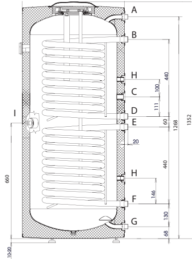
UBS 300 Sol indirekt HMV tároló méretei
