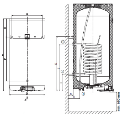
UBS 80 E W indirekt HMV tároló méretei
