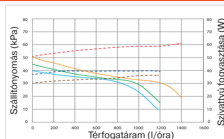
Szivattyú jelleggörbe
