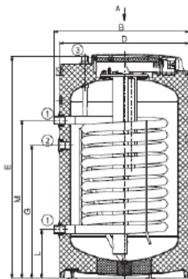
UBS 125 E indirekt HMV tároló méretei
