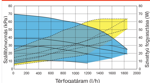
Szivattyú jelleggörbe
