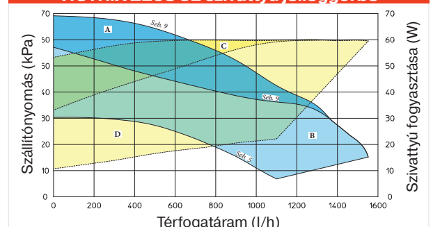
VICTRIX ZEUS 32 szivattyú jelleggörbe
