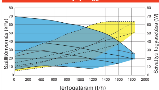
Szivattyú jelleggörbe
