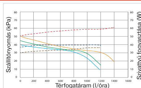
Szivattyú jelleggörbe
