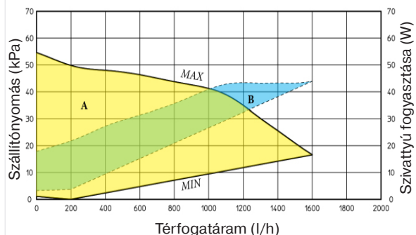
Szivattyúk jelleggörbéi
